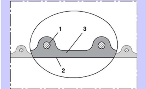
AIRDUCタイプホース 1. 壁内に螺旋状にしっかりと埋め込まれたステンレス鋼線 2. 恒久的帯電防止プレミアムエーテルポリウレタン 3. 肉厚:約1.4-1.5mm
